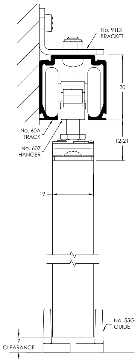
91LS BRACKETS
